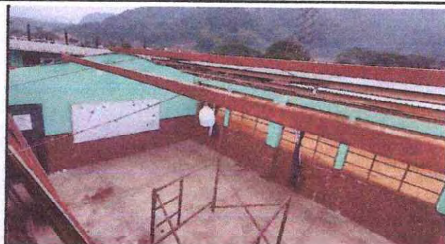
Foto 26: Sustitución de lámina por lámina troquelada aluzinc.
