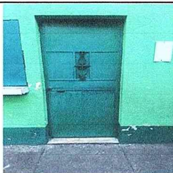
Foto 5: Puerta de metal deteriorada, Region 4.1 (Mantenimiento a estructura (lijado, cambio de tubo , cepillado, sujeciones, aplicación de pintura).
