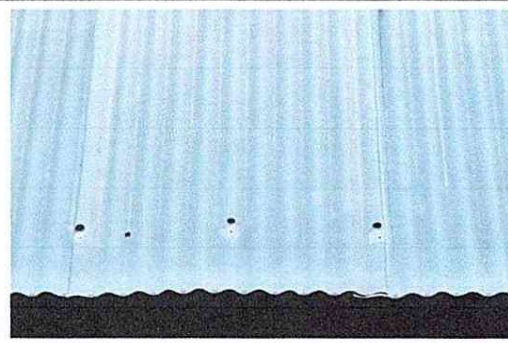
Foto 4: Elementos de fijación dañados, Region 1.3 (Sustitución de elementos de fijación).
