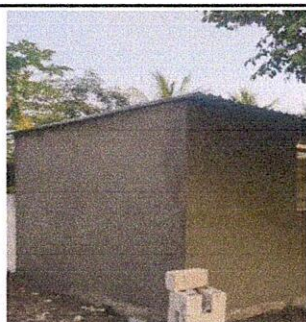
Foto 5: Muro, Region 15.1 (Reparación de muro perimetral de block) Region 21.2 (Cernido en muro)
