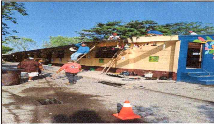
Foto1: 1. CUBIERTA DE LÁMINA 1.1 Sustitución de lámina, por lámina troquelada aluzinc calibre 26 1.2 Sustitución de capote de lámina para lámina troquelada 1.3 Sustitución de elementos de fijación
