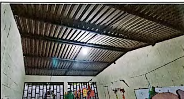
Foto 11: Suministro e instalación de sistema eléctrico iluminación y fuerza (incluye ducto y/o tubos de PVC, cajas octogonales, abrazaderas, cables, interruptores, tomacorrientes dobles, plafonera con foco ahorrador de alta potencia), finalizado al 100%.
