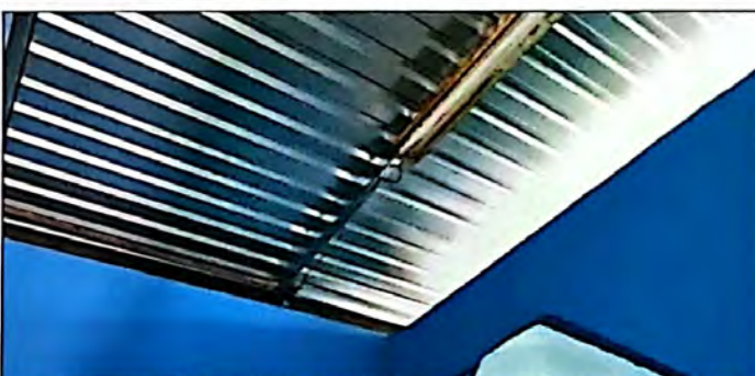
Foto 4: Suministro e instalación de lámina troquelada Aluzinc calibre 26 (incluye tornillos) en el módulo de baños. Finalizado al 100%.
