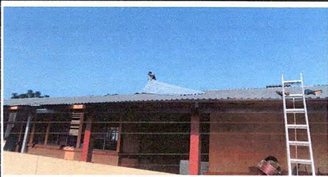
Foto 4: Colocación de lámina troquelada calibre 26 en los módulos 3 y 4 del segundo nivel.
