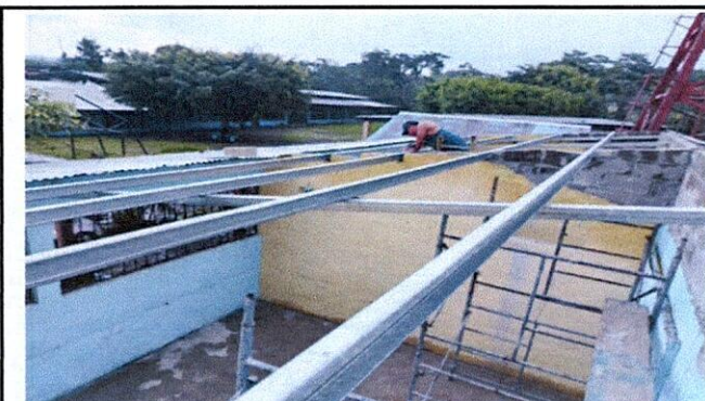
Foto 4: Instalación de estructura portante
