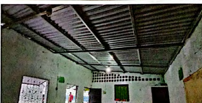
Foto 12: Cambio e instalación de lamina por lamina troquelada aluzinc calibre 26 (incluye pernos) en módulo de aula. Finalizado al 100%.
