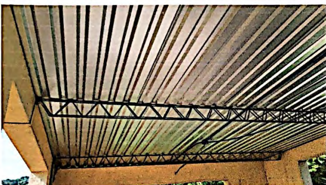
Foto 3: Cambio e instalación de lamina, por lamina troquelada aluzinc calibre 26 (incluye tornillos) en gradas del 1er. Módulo de aulas, finalizado al 100%.
