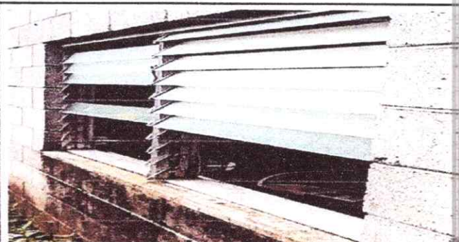
Foto 6: SUSTITUCIÓN DE BALCONES DE METAL LADO DE ATRÁS
