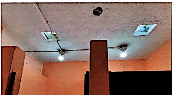
Foto 5: Reparación de circuito de iluminación (incluye ducto o tubo PVC, abrazaderas, cajas octogonales, cables, interruptores, plafonera con foco ahorrador de alta potencia. Finalizada al 100%
