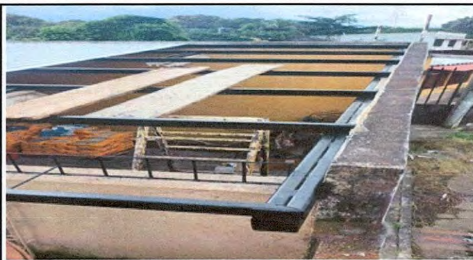
FOTO:2 Sustitución de lámina, por lámina Troquelada, Aluzinc Calibre 26. 50 %.
