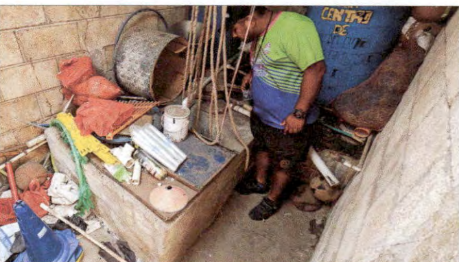
Foto 11: Se detecta la necesidad de darle mantenimiento al pozo así como el cambio e instalación de bomba sumergible 1hp incluye accesorios y conexión de tubería.
