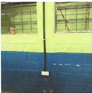
Foto 3: Sustitucion de sistema electrico salon 12 finalizado
