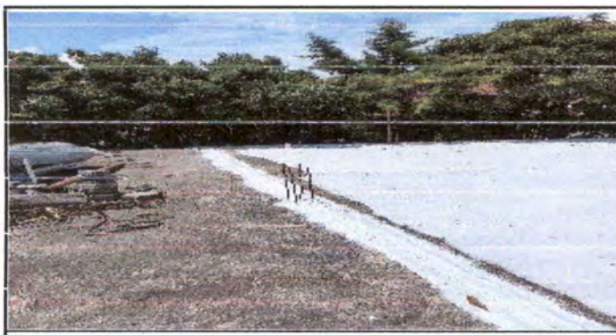
Foto 11: Situación de terraza durante la aplicación del impermeabilizante.
