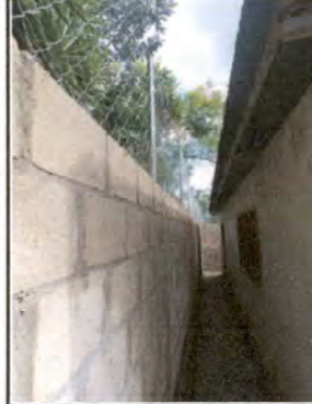
Foto 8: Estado final del muro perimetral de block con tubo hg y malla galvanizada
