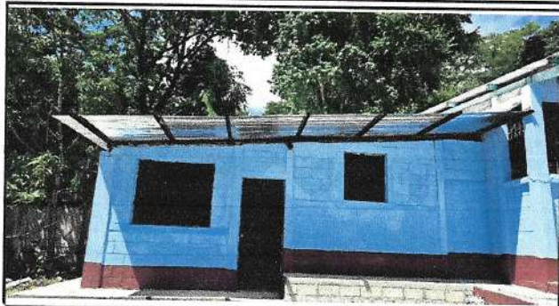
Foto 1: Remozamiento de muros de la cocina, sustitución de tela maya por muro de block
