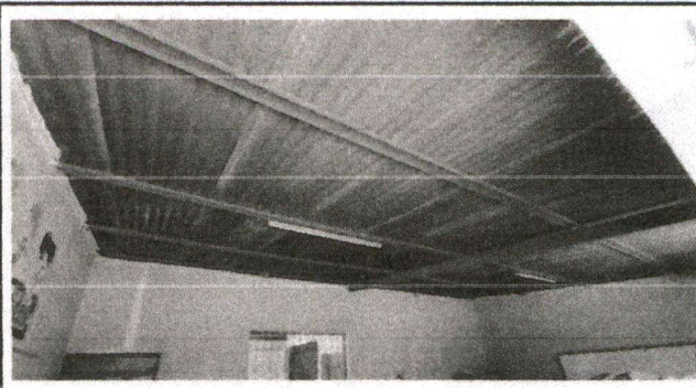
Foto 2: SUSTITUCION E INSTALACION DE LAMINAS CON COSTANERAS DE METAL
