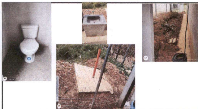
Foto 3: REPARACIÓN DE RED DE DRENAJES Y AGUA: REFORZAMIENTO DE FOSA SÉPTICA, SUSTITUCIÓN DE TUBERÍA PVC LINEA PRINCIPAL AGUAS NEGRAS (3 PULGADAS), RED DE AGUA ENTUBADA, (SUSTITUCIÓN DE TUBERÍA PVC LINEA PRINCIPAL Y SUS ACCESORIOS INSTALACIÓN INCLUIDA).
