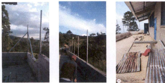
Foto1: MURO PERIMETRAL: REPARACIÓN DE MURO PERIMETRAL DE BLOCK CON TUBO HG Y MALLA GALVANIZADA (125 M2).
