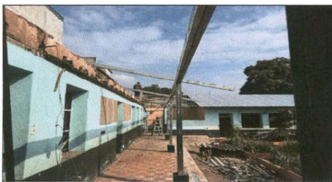
Foto 5: INSTALACION DE COSTANERA DE METAL EN CORREDOR
