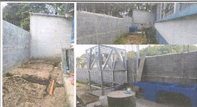
Foto 3: Instalación de pilas, con drenaje, construcción de galera y estructura de metal para sostener el tinaco.
