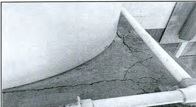
Foto 3: El peso del tinaco esta deteoriando la plancha en la que se encuentra
