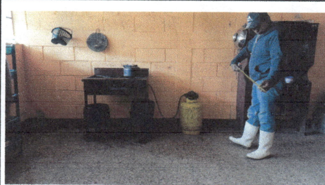
Foto 2: Instalación de estufa rural (completa).
