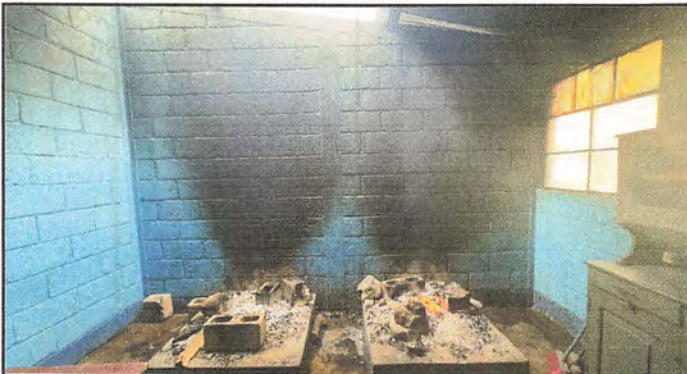
Foto 3: Construcción de 3 chimeneas de metal con sus respectivos extractores de humo.
