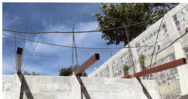
Renglon 2: vigas de costanera para sujetar las láminas del techado.
