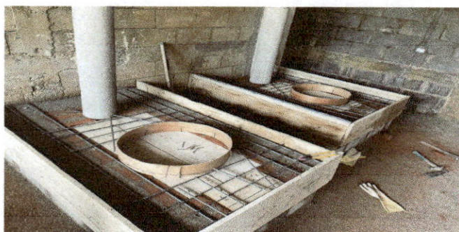
Renglón 8: reparación de estufas rurales para mejorar la preparación de alimentos.
