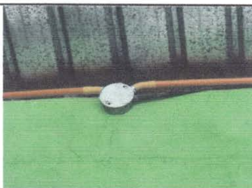
Foto 6: Cambio de ductos y cajas octogonales.
