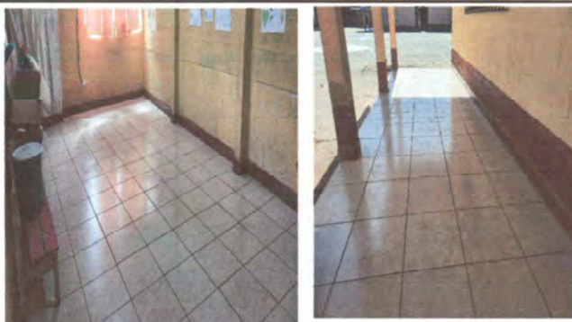
Foto 3: colocación de piso de aula y corredor No. 14 solitaria
