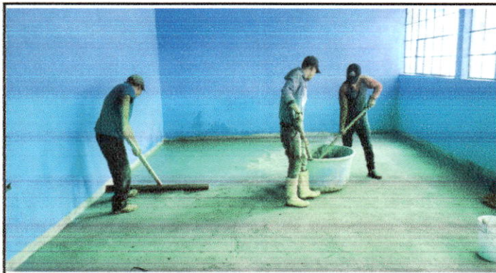
Foto 9: Preparación de base para colocación de piso
