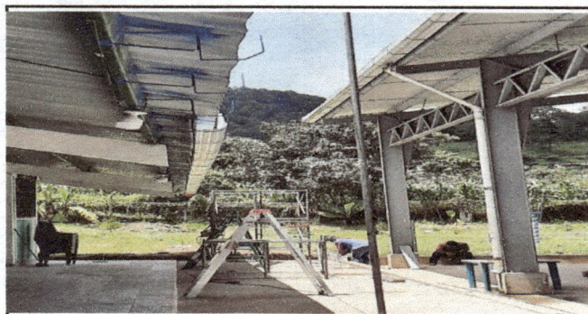
Colocacion de canales en frente de aulas y direccion.
