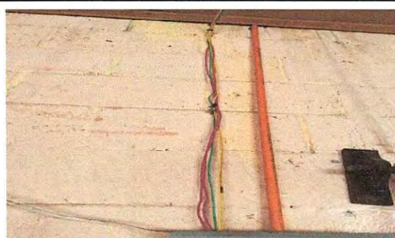
Foto 14 : Sustrucción de ducto eléctrico + accesorios
