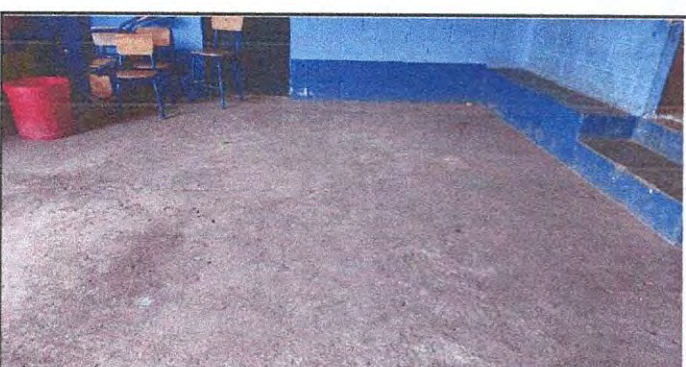
Foto 6: Colocación de piso cerámico enfrente de cocina
