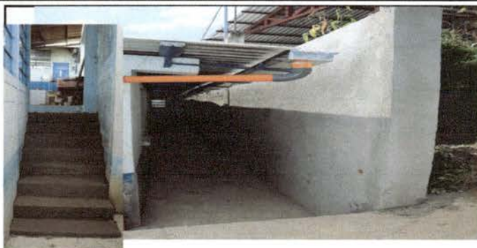
Foto 2: Mejoramiento de cuneta de Cuneta exterior, cernido gris en la parte de atrás de los salones, muro de block y construcción de gradas de concreto
