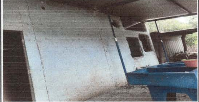
Foto 2: esta pared que sostiene la cumbrera y todo el techo de la cocina se demolera y se colocara un tuvo de 6x2 de metal con sus refuerzos
