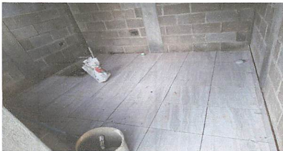
Foto 11: Instalación de cajas eléctricas
